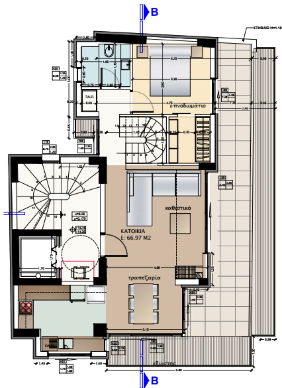
Κάτοψη 5ου ορόφου Μεζονέτας Κάτοψη Μεζονέτας-5ου-6ου ορόφου
