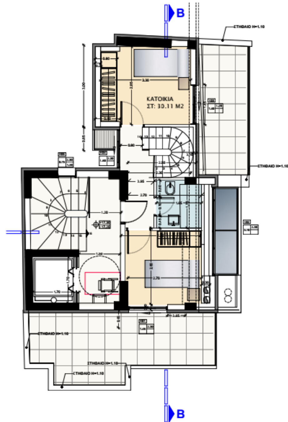
Κάτοψη 6ου ορόφου Μεζονέτας
