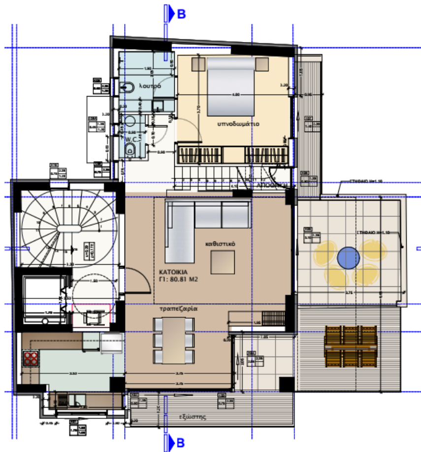
Κάτοψη 3ου ορόφου Μεζονέτας Κάτοψη Μεζονέτας-3ου-4ου ορόφου
