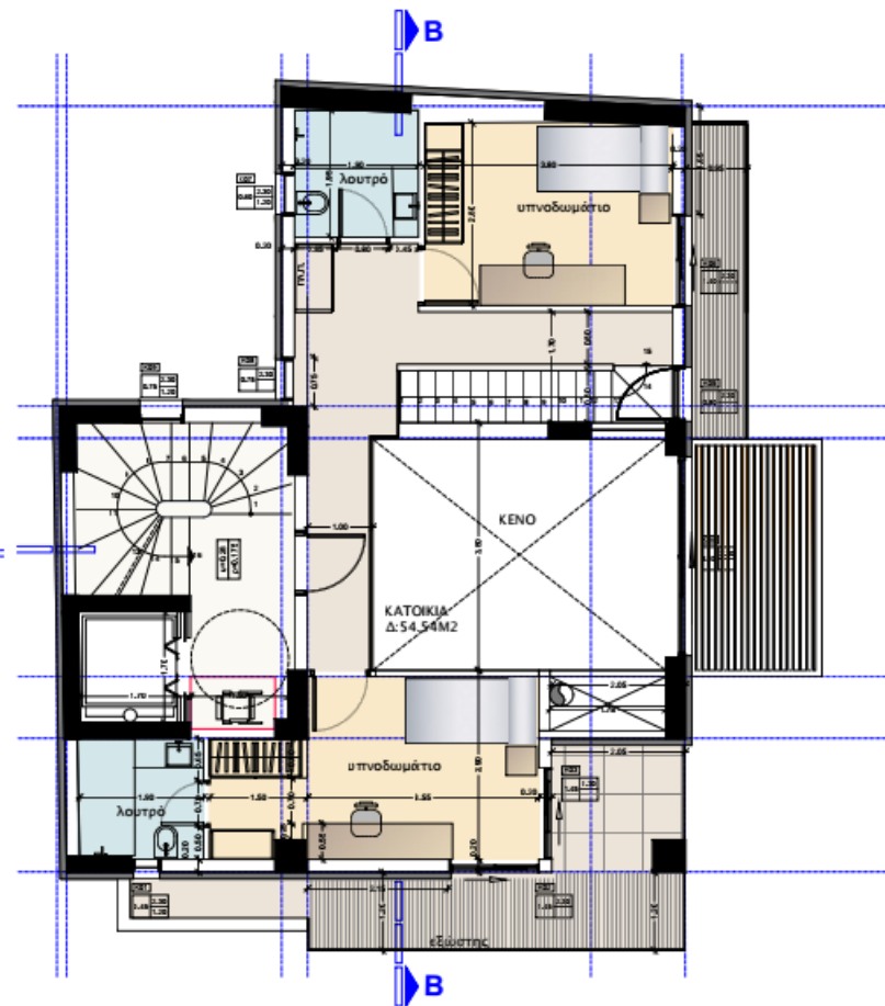
Κάτοψη 4ου ορόφου Μεζονέτας
