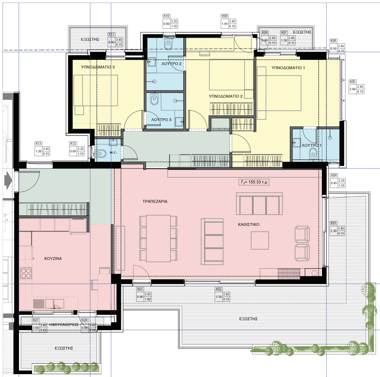
ΚΑΤΟΦΗ ΔΙΑΜΕΡΙΣΜΑΤΟΣ Γ3 ΚΛΙΜ. 1:100
